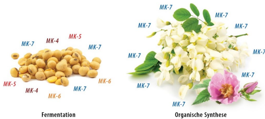
Abb. 2: Gebildete Vitamin K2-Formen nach Herstellung durch Fermentation und organische Synthese
