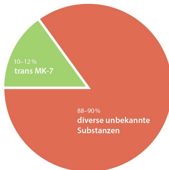
Abb. 3: Anteil an trans MK-7 und unbekannten Substanzen in Vitamin-K2-Rohstoffen aus China
