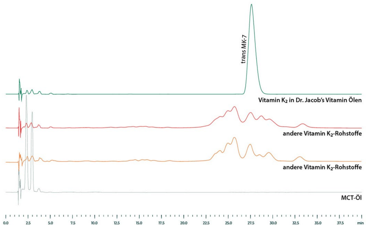
Abb. 4: UPLC-Analyse verschiedener Vitamin K2-Rohstoffe
